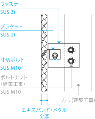
断面
